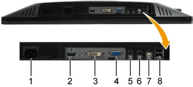
下面外觀
